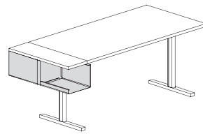
Marsupio laterale aperto/chiuso Items holder open / closed Porte objets ouvert / fermé L. 24 - P. 80 - H. 25
