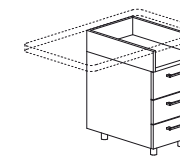
Modulo cassetiera portante a tre cassetti Fixed pedestal with 3 drawers Caisson fixe avec 3 tiroirs L. 42 - P. 59 - H. 70
