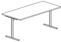
Scrivanie Desk Bureau L. 140/160/180/200 - P. 80 - H. 74
