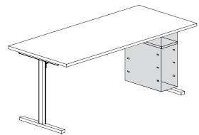
Porta Pc appeso in acciaio CPU holder Porte UC L. 26 - P. 50 - H. 57,6
