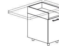
Modulo anta destra/sinistra portante RH/LH hinged door fixed side cabinet Porte gauche/droite armoire latéral fixe L. 42 - P. 59 - H. 70
